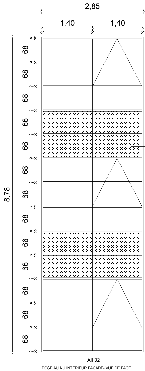
ME03 ENSEMBLE MENUISÉ AVEC OUVRANTS CACHÉS
