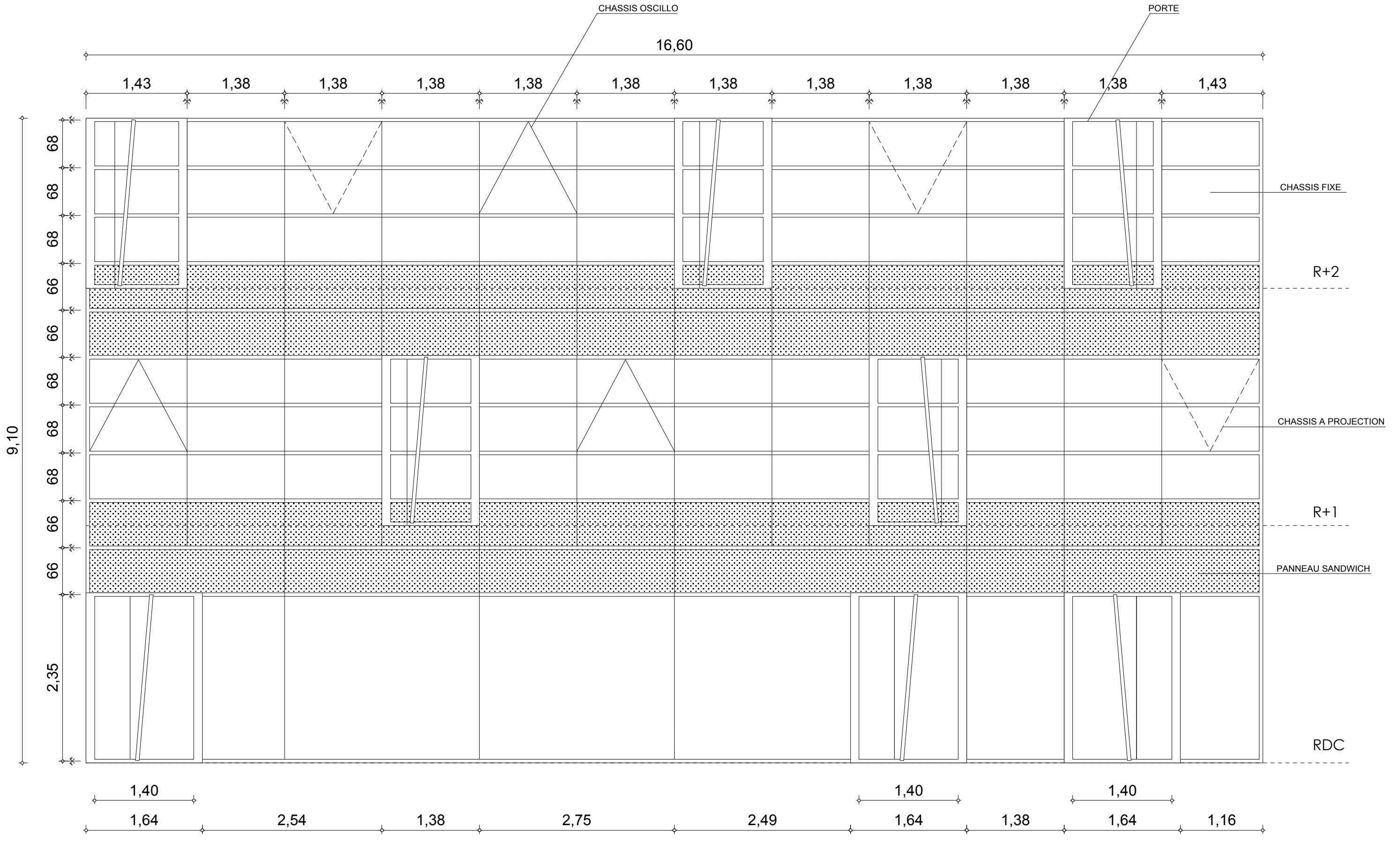
ME05 ENSEMBLE MENUISÉ AVEC OUVRANTS CACHÉS OSCILLO ET A PROJECTION + PORTES
