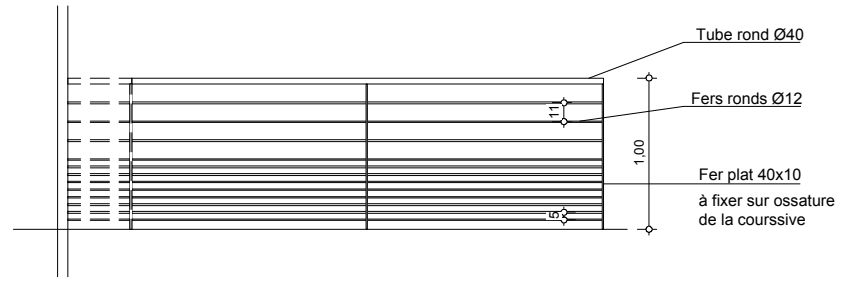
GARDE CORPS
